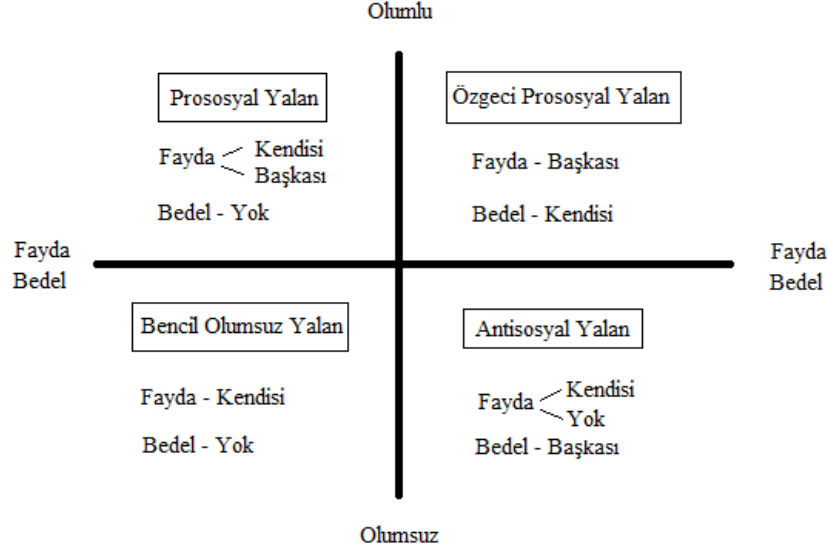
Şekil 1. Yalan Sınıflandırması
