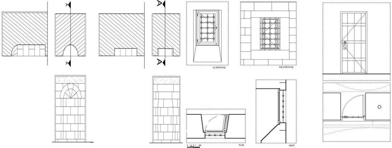
Şekil 52,53. Hüsrev Paşa Külliyesi Çifte Hamamı Kadınlar Bölümü Mihrap ve Niş Plan, Kesit Detayları (Ş. Öztürk)
