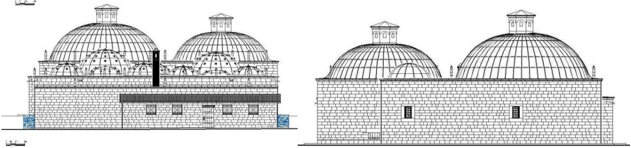
Şekil 62,63. Hüsrev Paşa Külliyesi Çifte Hamamı Doğu ve Batı Cepheleri (Ş. Öztürk)
