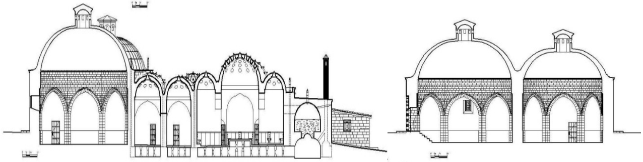
Şekil 73,74. Hüsrev Paşa Külliyesi Çifte Hamamı A-A ve B-B Kesiti (Ş. Öztürk)
