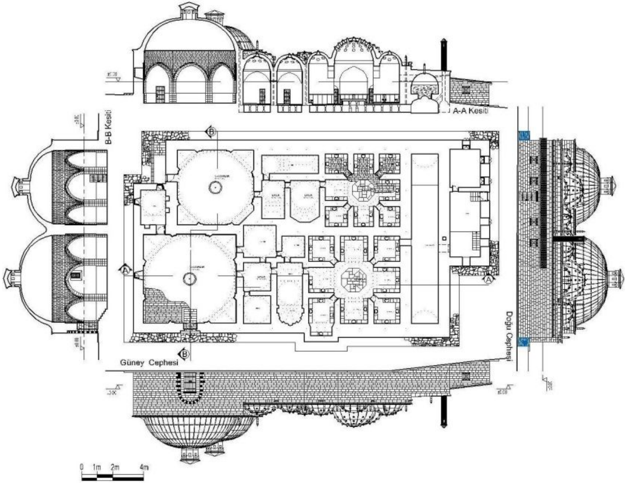
Şekil 8. Hüseyin Paşa Külliyesi Çifte Hamam Planı, Kesit ve Cepheleri (Ş. Öztürk)
