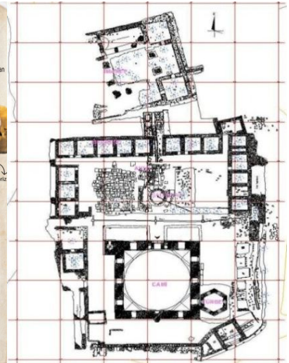
Şekil 7. H.P.K Rölöve Vaziyet Planı (Ş. Öztürk)
