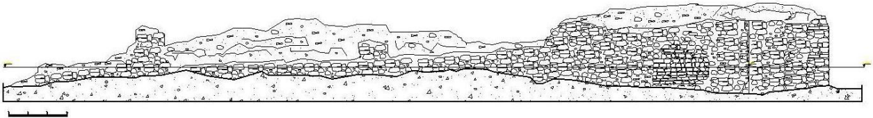
Şekil 46. Hüsrev Paşa Külliyesi Çifte Hamam Kuzey Cephe Rölövesi (Ş. Öztürk)
