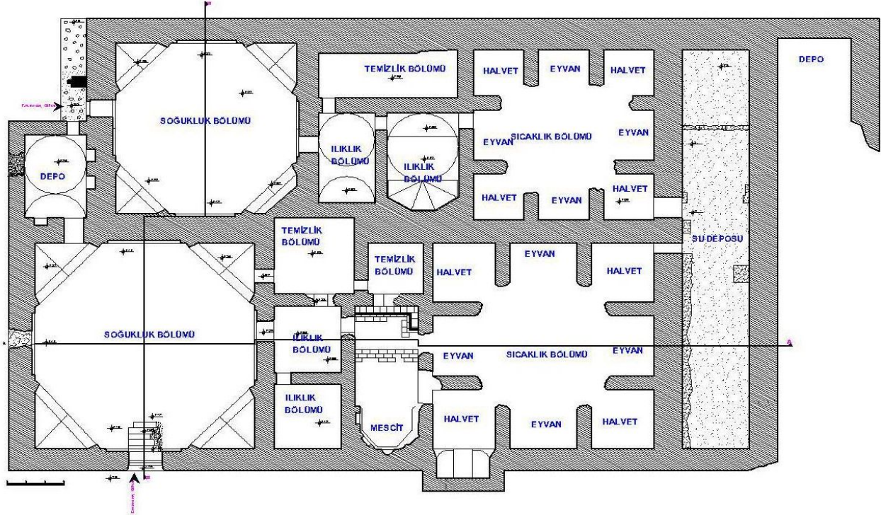
Şekil 39. Hüsrev Paşa Külliyesi Çifte Hamam Rölöve Planı (Ş. Öztürk)
