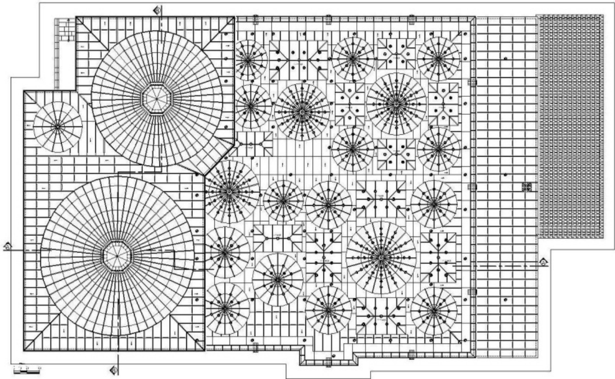
Şekil 70. Hüseyin Paşa Külliyesi Çifte Hamamı Örtü Planı (Ş. Öztürk)
