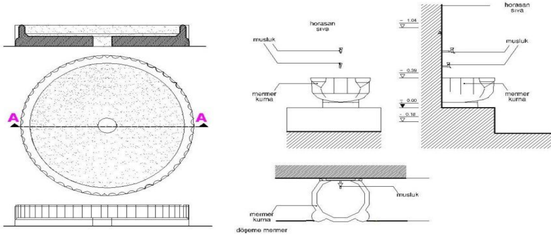
Şekil 55,56. Çifte Hamam Havuz, Kürne, Künk (Pöhrék), Tuğla ve Zemin Kanal Detayları (Ş. Öztürk)
