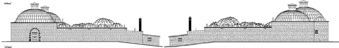
Şekil 66,67. Hüsrev Paşa Külliyesi Çifte Hamamı Güney ve Kuzey Cepheleri (Ş. Öztürk)
