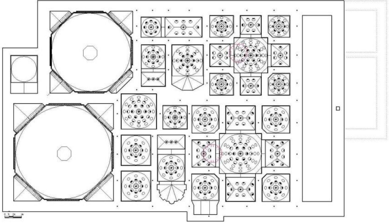
Şekil 54. Hüsrev Paşa Külliyesi Çifte Hamamı Tavan Planı (Ş. Öztürk)
