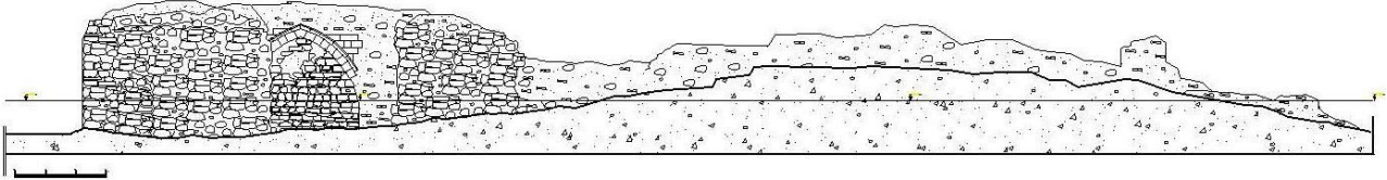
Şekil 45. Hüsrev Paşa Külliyesi Çifte Hamam Güney Cephe Rölövesi (Ş. Öztürk)
