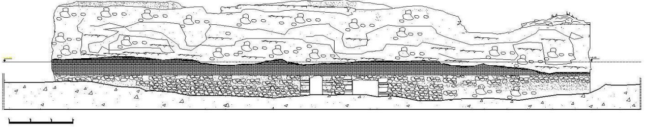
Şekil 44. Hüsrev Paşa Külliyesi Çifte Hamam Doğu Cephe Rölövesi (Ş. Öztürk)
