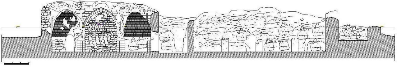
Şekil 41. Hüsrev Paşa Külliyesi Çifte Hamam A-A Kesit Rölövesi (Ş. Öztürk)
