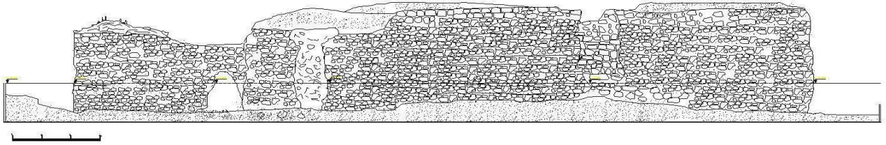
Şekil 43. Hüsrev Paşa Külliyesi Çifte Hamam Batı Cephe Rölövesi (Ş. Öztürk)
