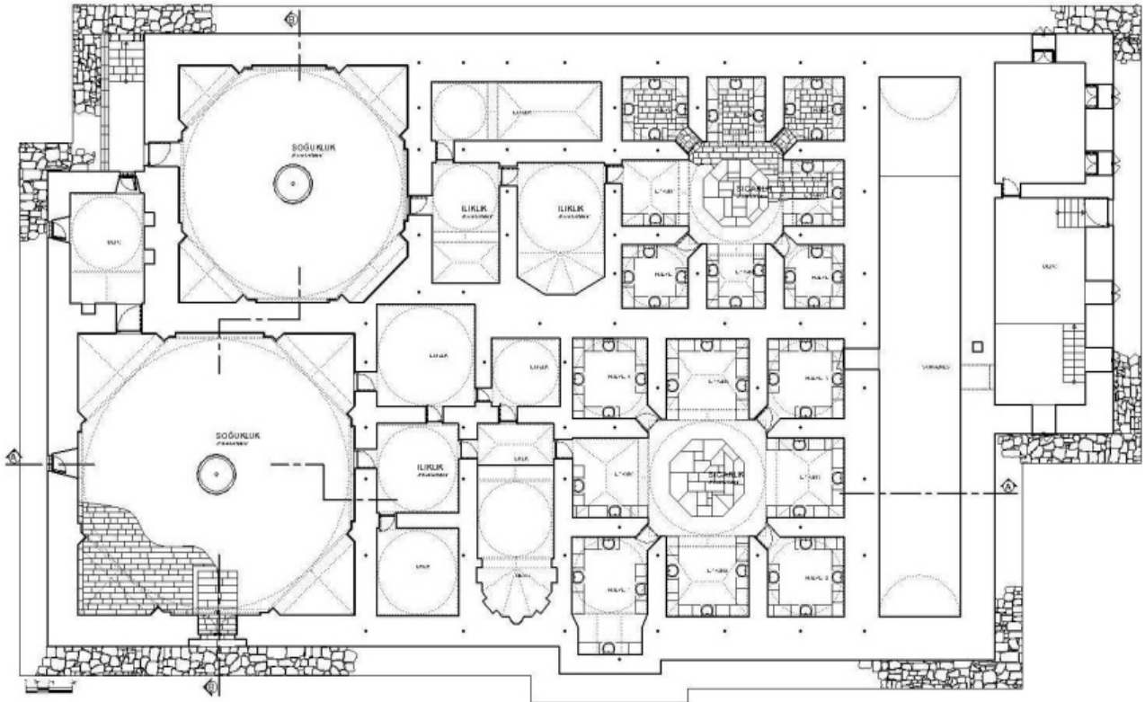
Şekil 51. Hüsrev Paşa Külliyesi Çifte Hamamı Planı (Ş. Öztürk)
