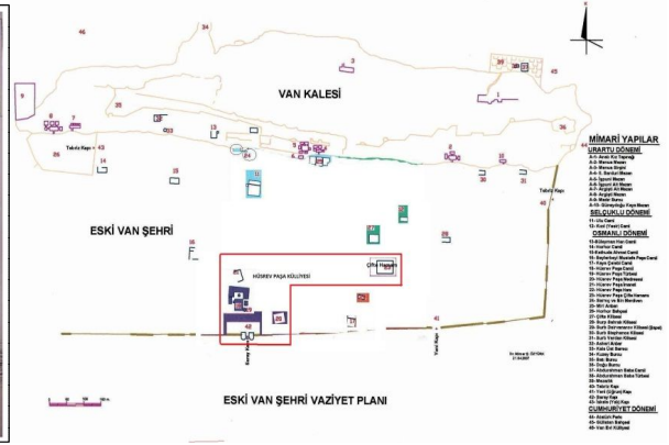
Şekil 2. Van Kalesi-Eski Van Şehir Vaziyet Planı (Ş. Öztürk)
