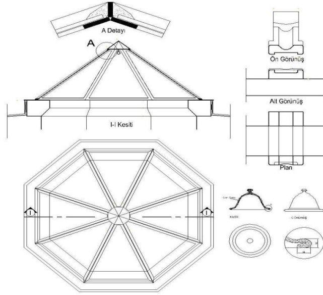
Şekil 71,72. Hüsrev Paşa Külliyesi Çifte Hamam Fenerlik, Çörten ve Cam Fanus Detayları (Ş. Öztürk)
