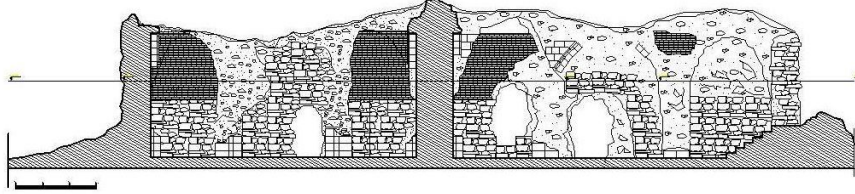
Şekil 42. Hüsrev Paşa Külliyesi Çifte Hamam B-B Kesit Rölövesi (Ş. Öztürk)
