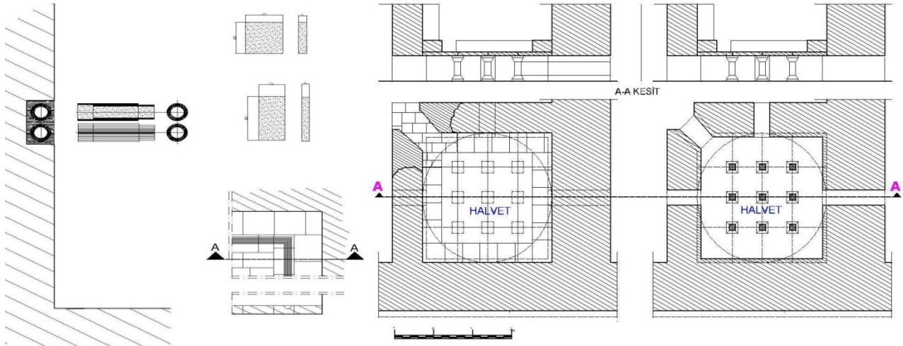
Şekil 75,76. Hüsrev Paşa Külliyesi Çifte Hamam Tuğla, Künk, Zemin Su Kanalı ve Halvet Plan-Kesit Detayları (Ş. Öztürk)
