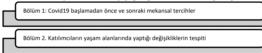
Şekil 3. Anket aşamaları
